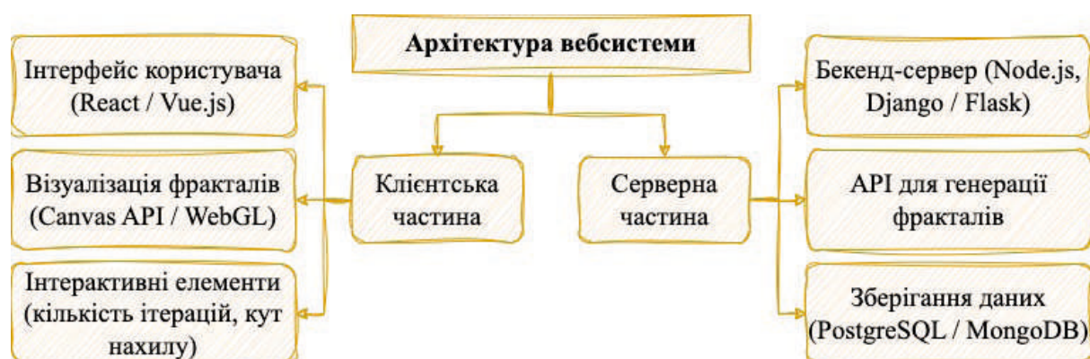
Рис. 1. Архітектура вебсистеми
