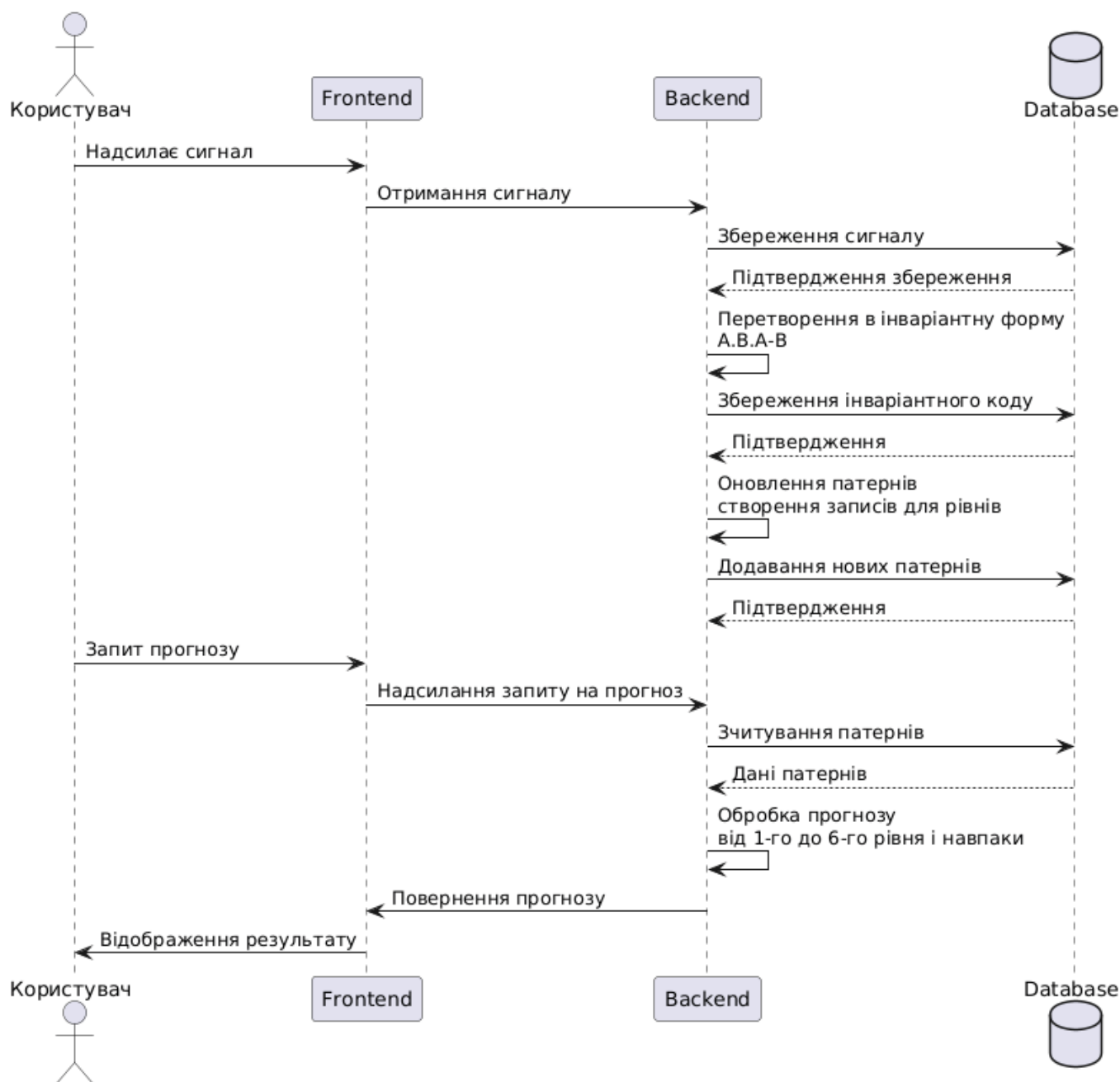
Рис. 1. Діаграма послідовності
