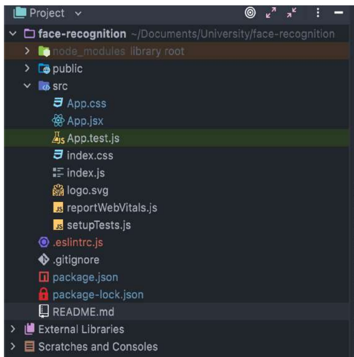
Рис. 1. Структура проекту
